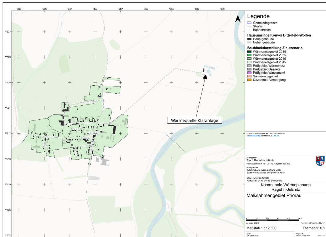
Abbildung 32: Karte zur Eignungsprüfung Wärmenetzgebiet Piorau
