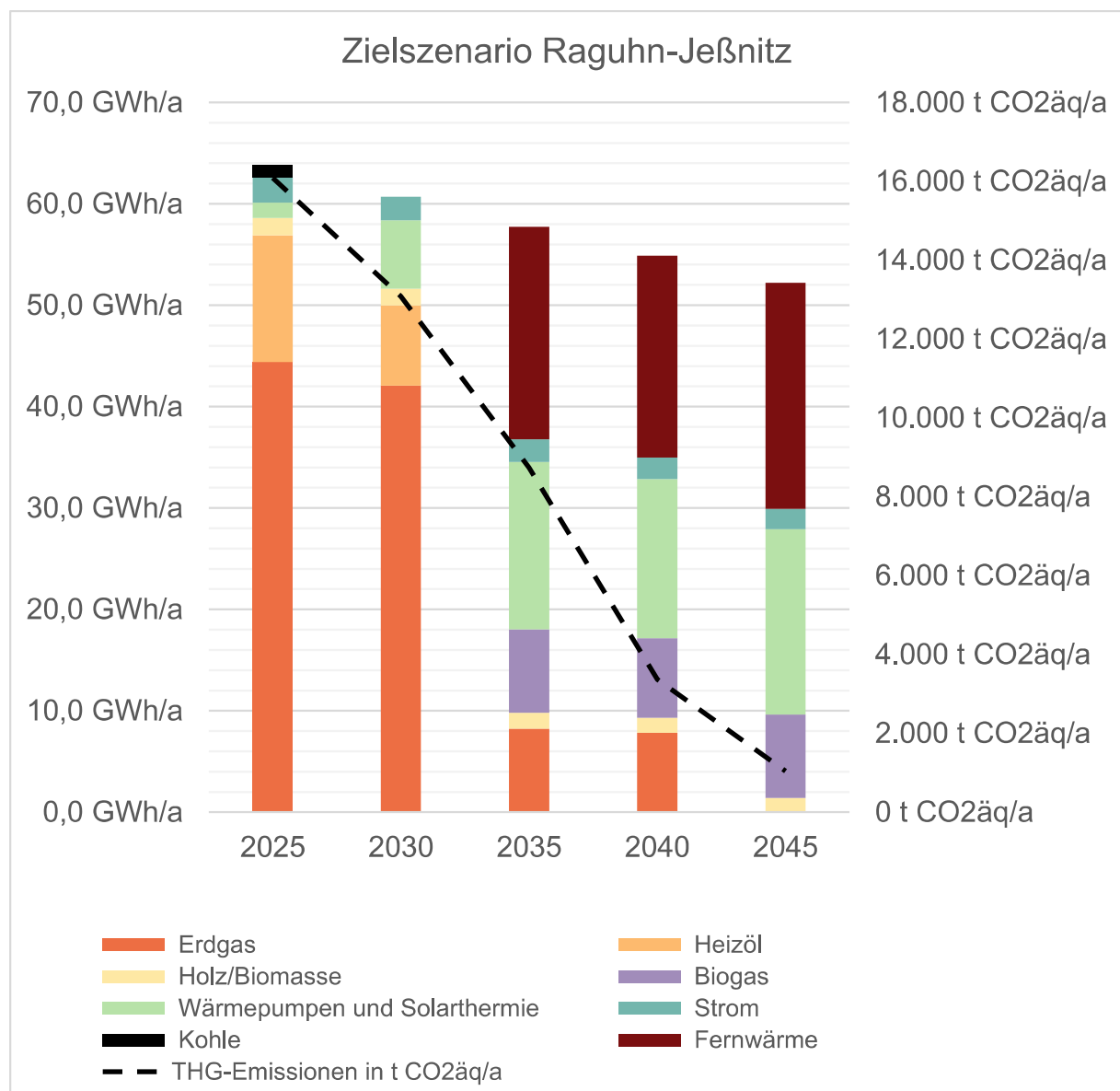
Abbildung 28: Entwicklung der Beheizungsstruktur und der Treibhausgasemissionen im Zielszenario
