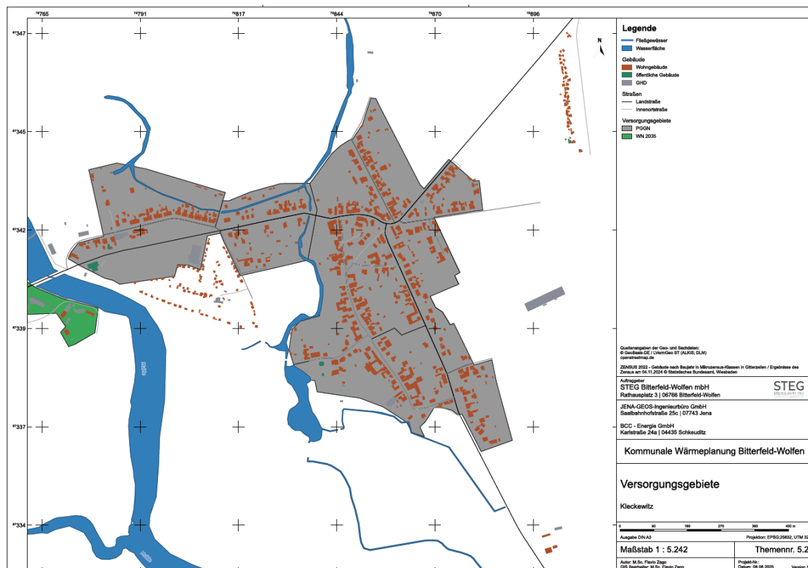
Abbildung 35: Prüfgebiet Gasnetz Kleckwitz
